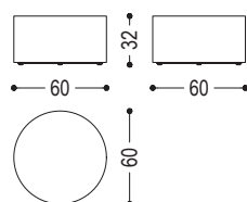
NATURA-ECO 1 CM. Ø 60 - H. 32
