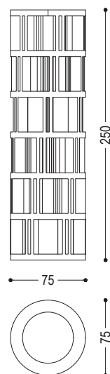
TORRE LIGNEA CM: Ø 75 · H. 250
