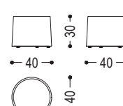
LEGNO VIVO 5 CM: Ø 40 · H. 30
